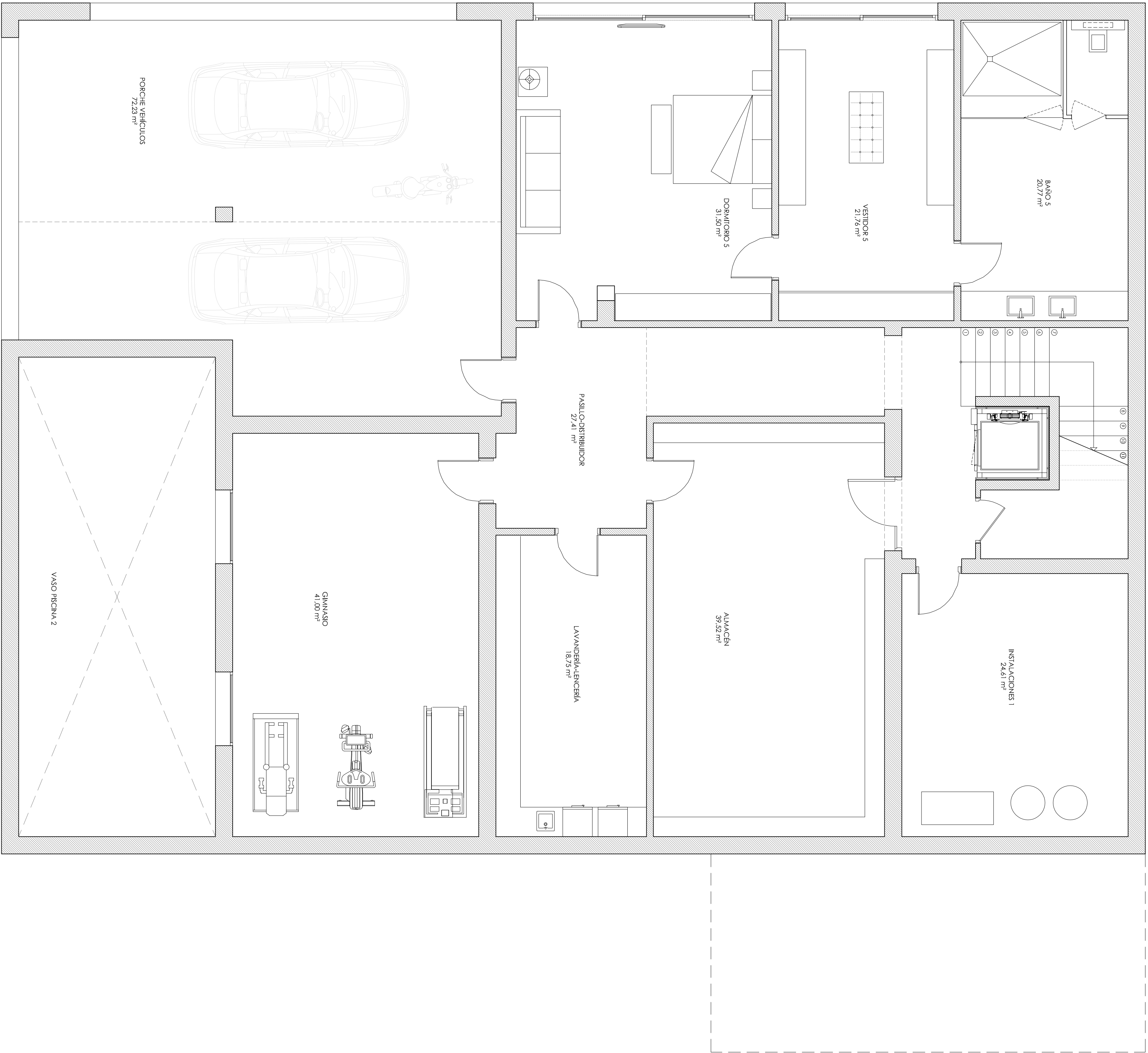
PLANTA SÓTANO (Nivel +90,70 m)
